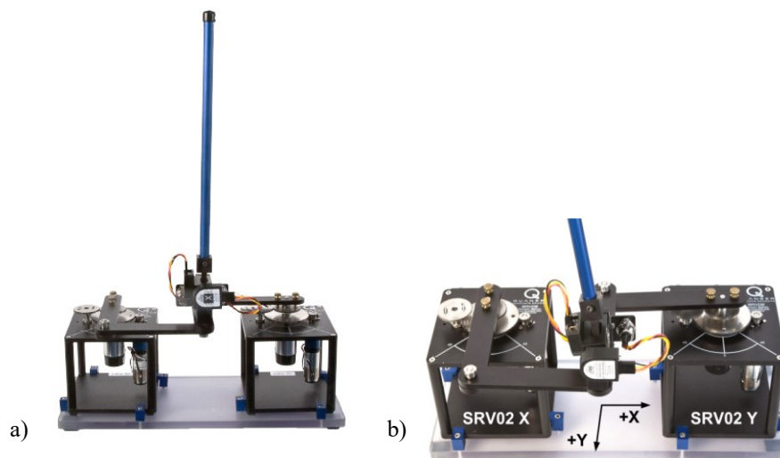
Fig. 1: The test stand [Quanser 2012]
